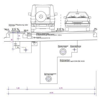
Regelquerschnitt Straße:
